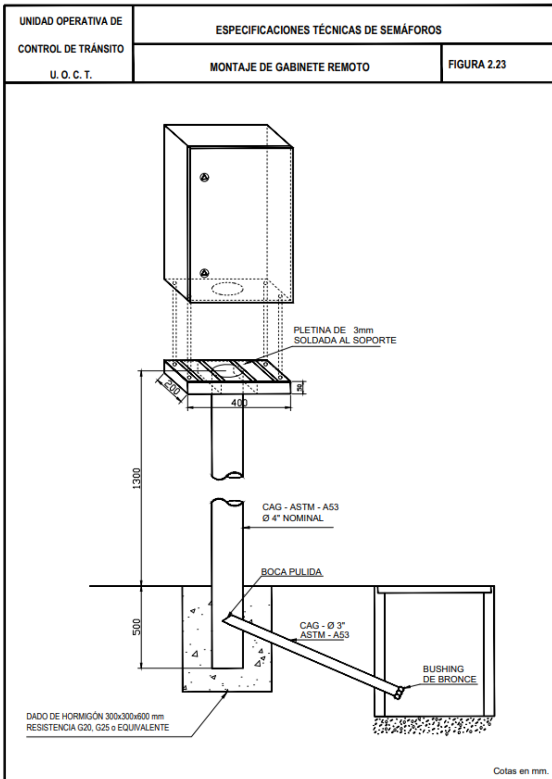
Figura 2. 23 Montaje de gabinete remoto
