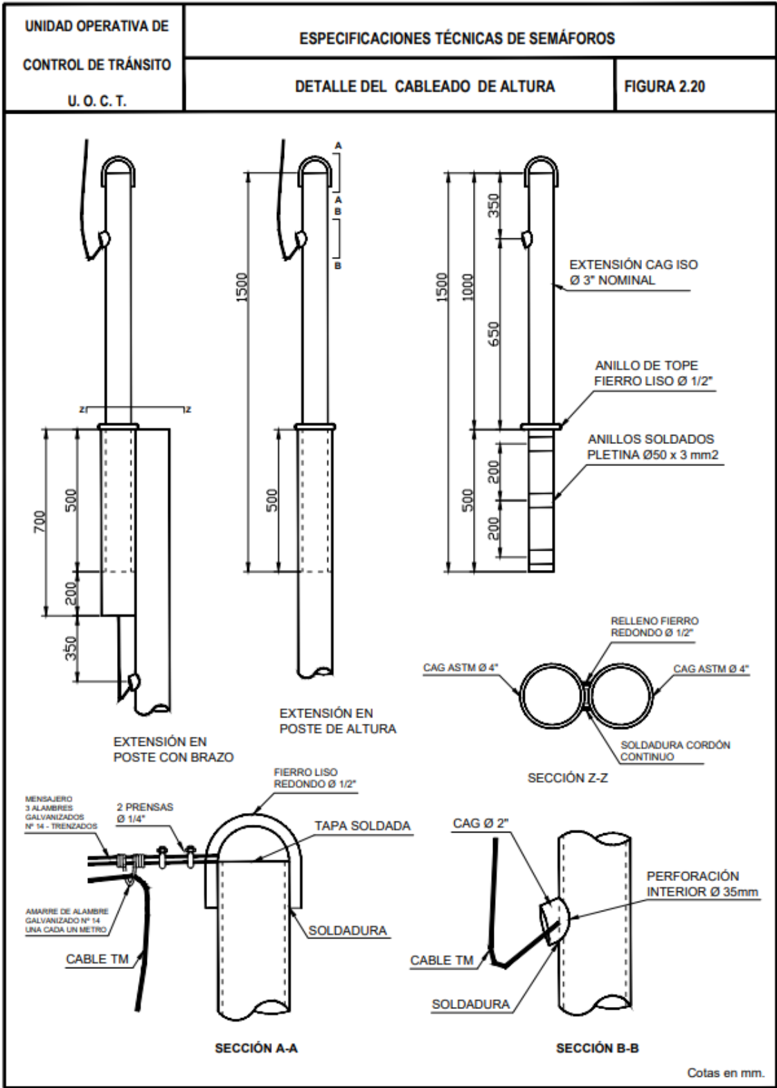
Figura 2. 20 Detalle del cableado de altura
