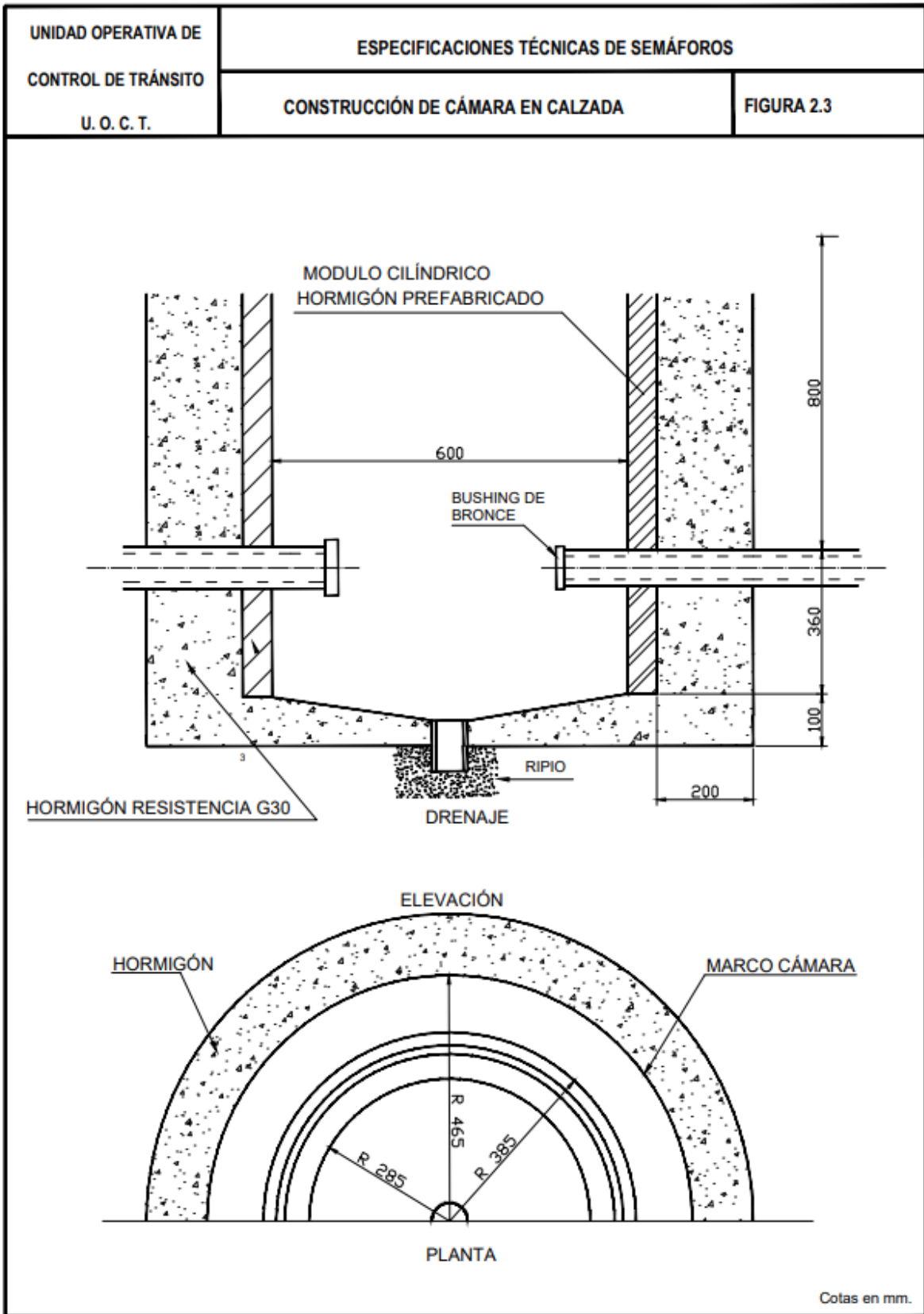
Figura 2. 3 Construcción de cámara en calzada
