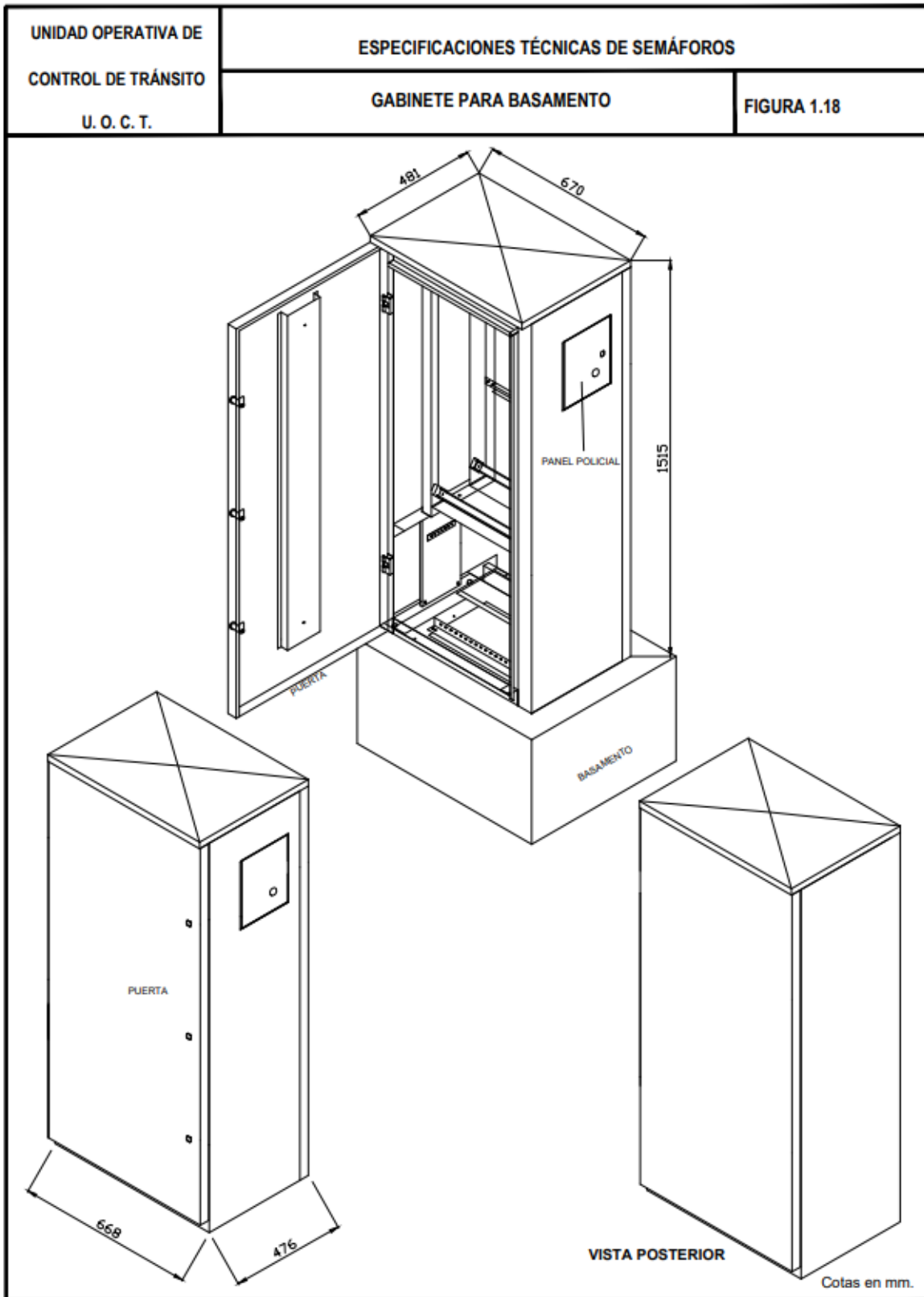
Figura 1. 18 Gabinete para basamento
