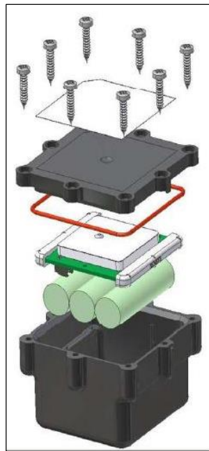
Figura 2. 32 Vista en explosión del Sensor
