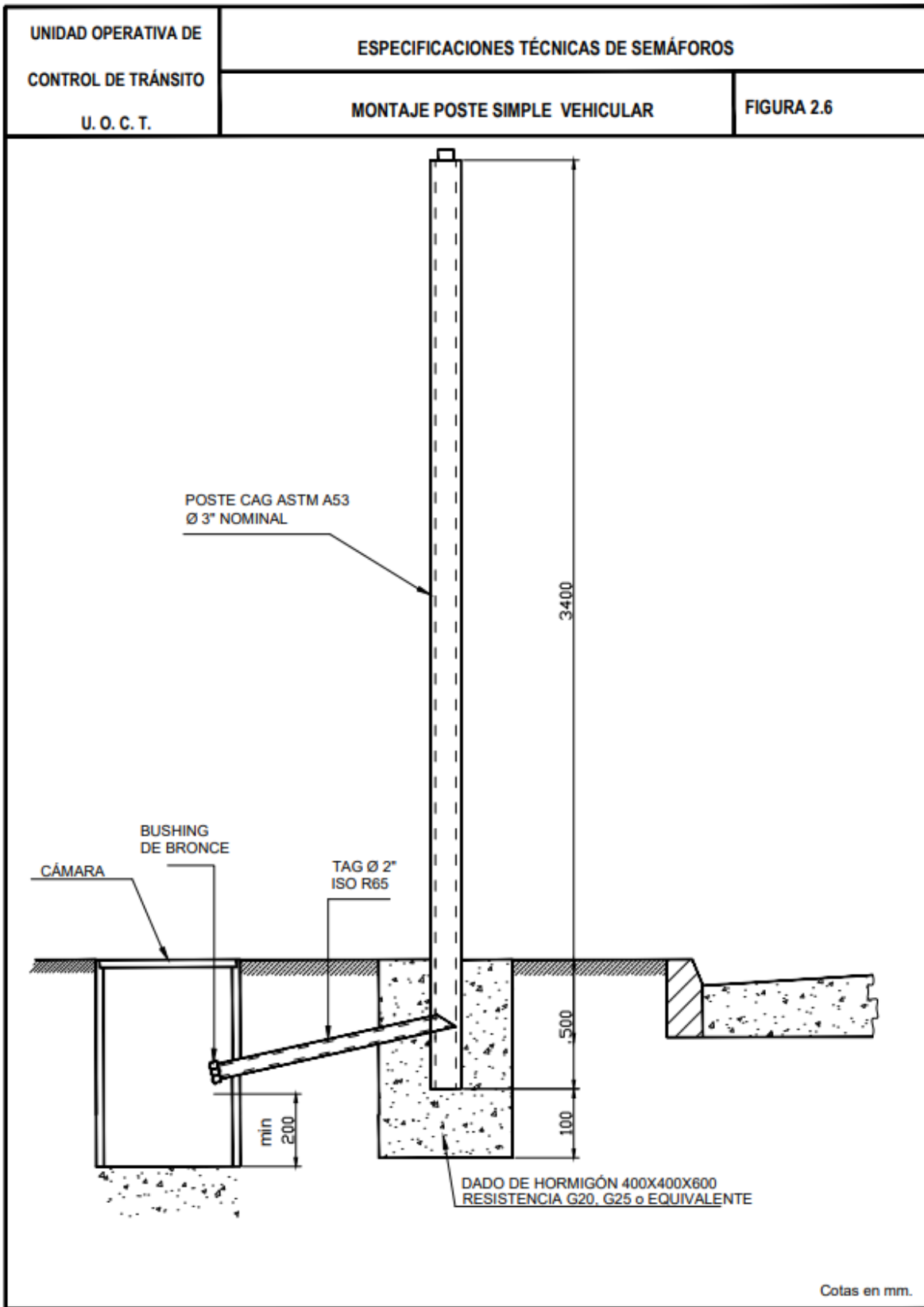
Figura 2. 6 Montaje poste simple vehicular
