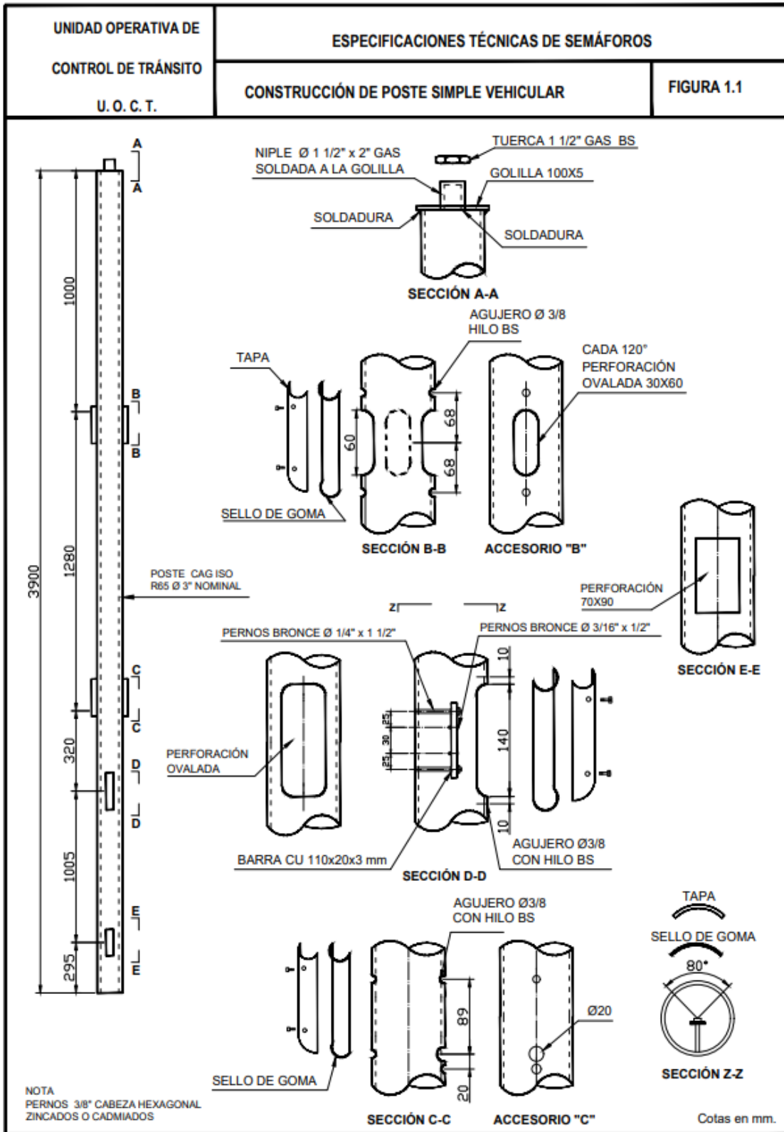
Figura 1. 1 Construcción de poste simple vehicular
