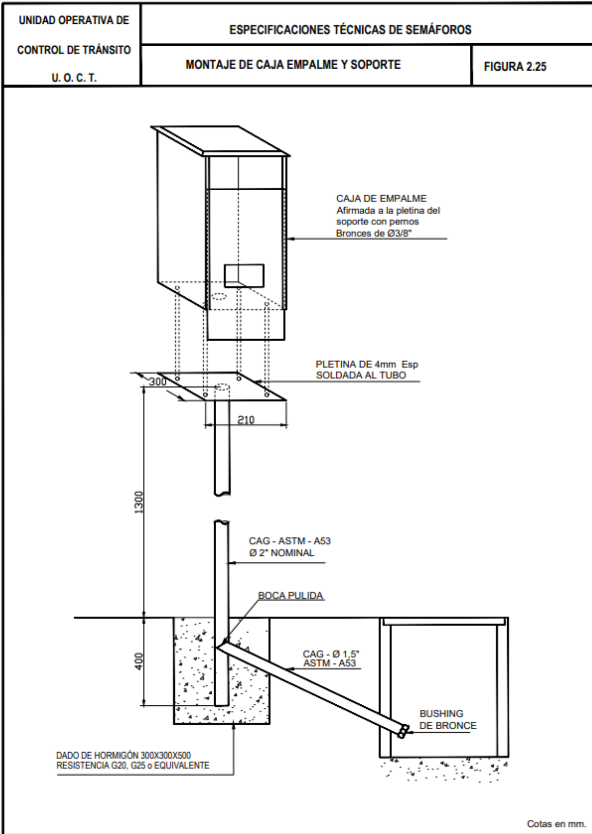
Figura 2. 25 Montaje de caja empalme y soporte
