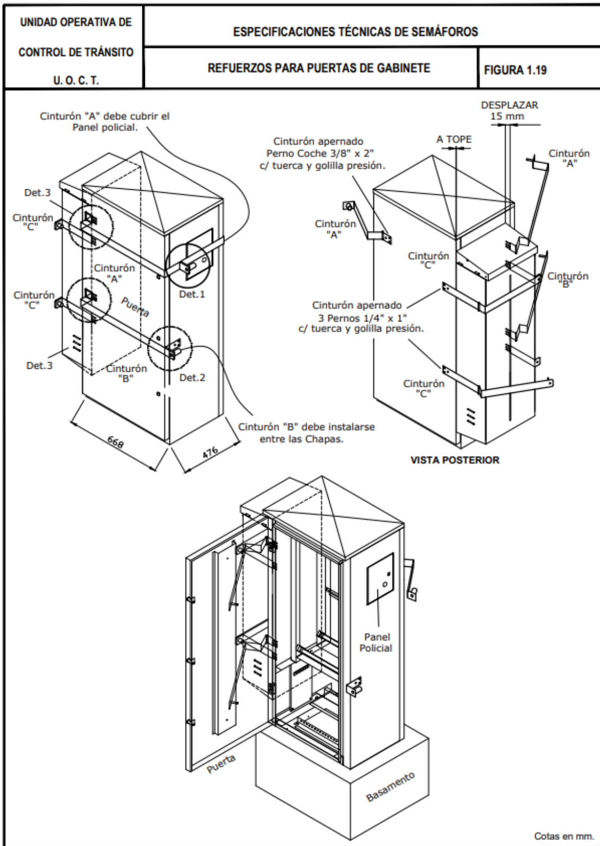
Figura 1. 19 Refuerzos para puertas de gabinetes
