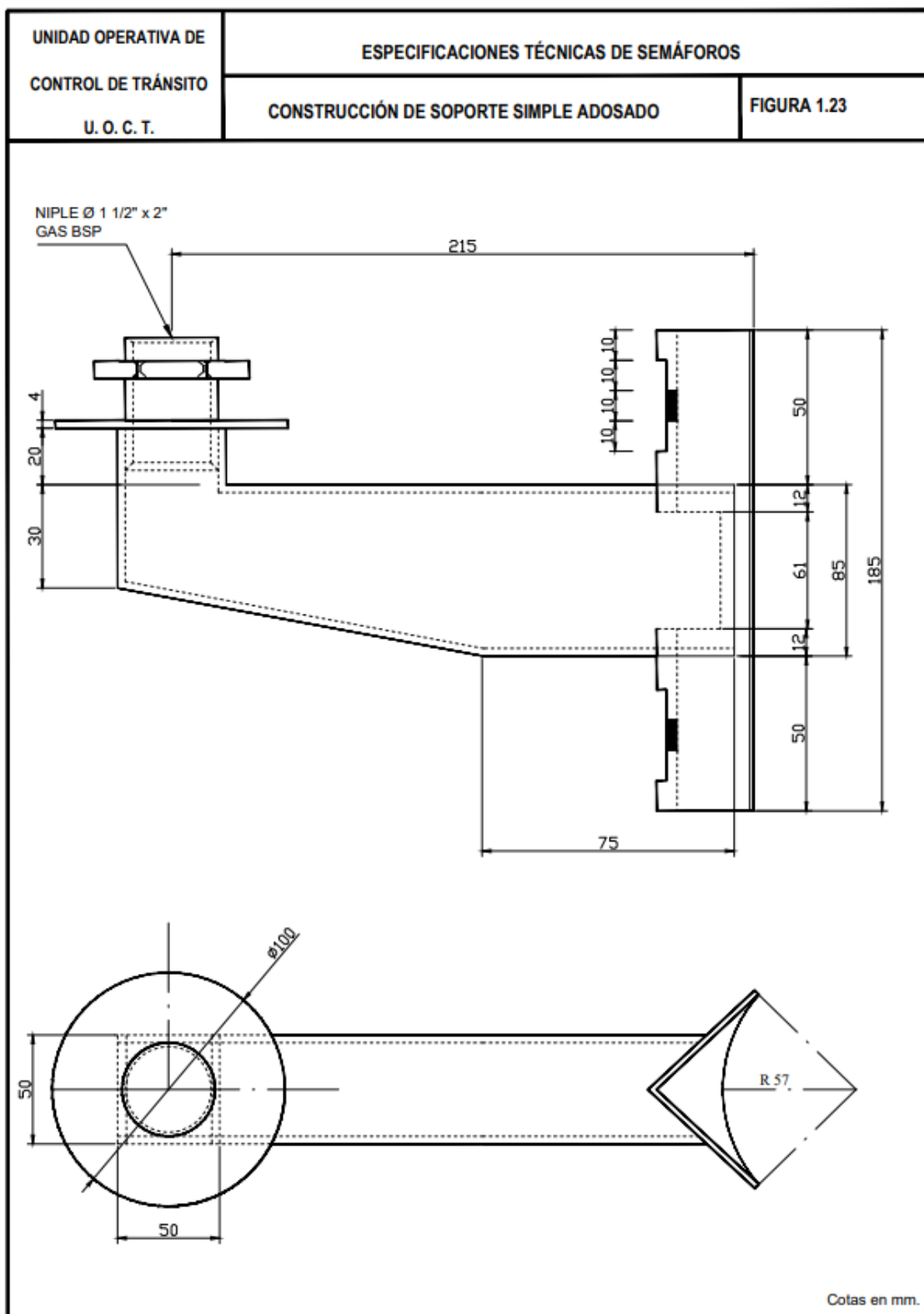
Figura 1. 23 Construcción de soporte simple adosado
