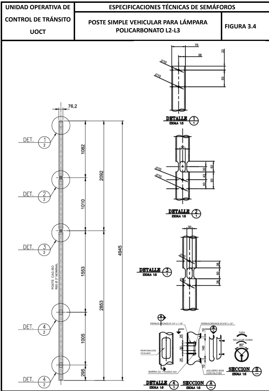
Figura 3. 4 Poste Simple Vehicular para Lámpara de Policarbonato L2-L3
