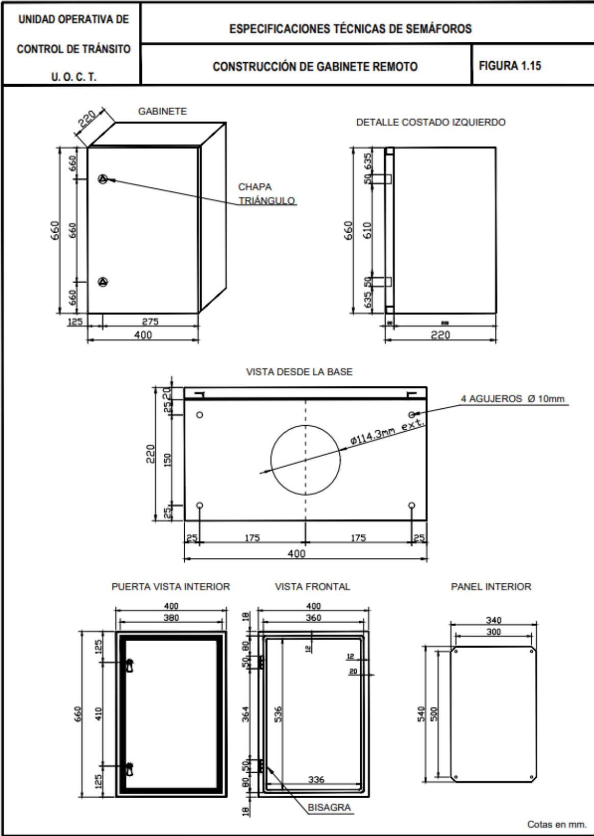
Figura 1. 15 Construcción de gabinete remoto
