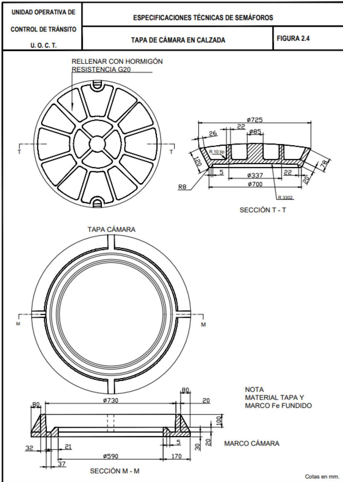
Figura 2. 4 Tapa de cámara en calzada
