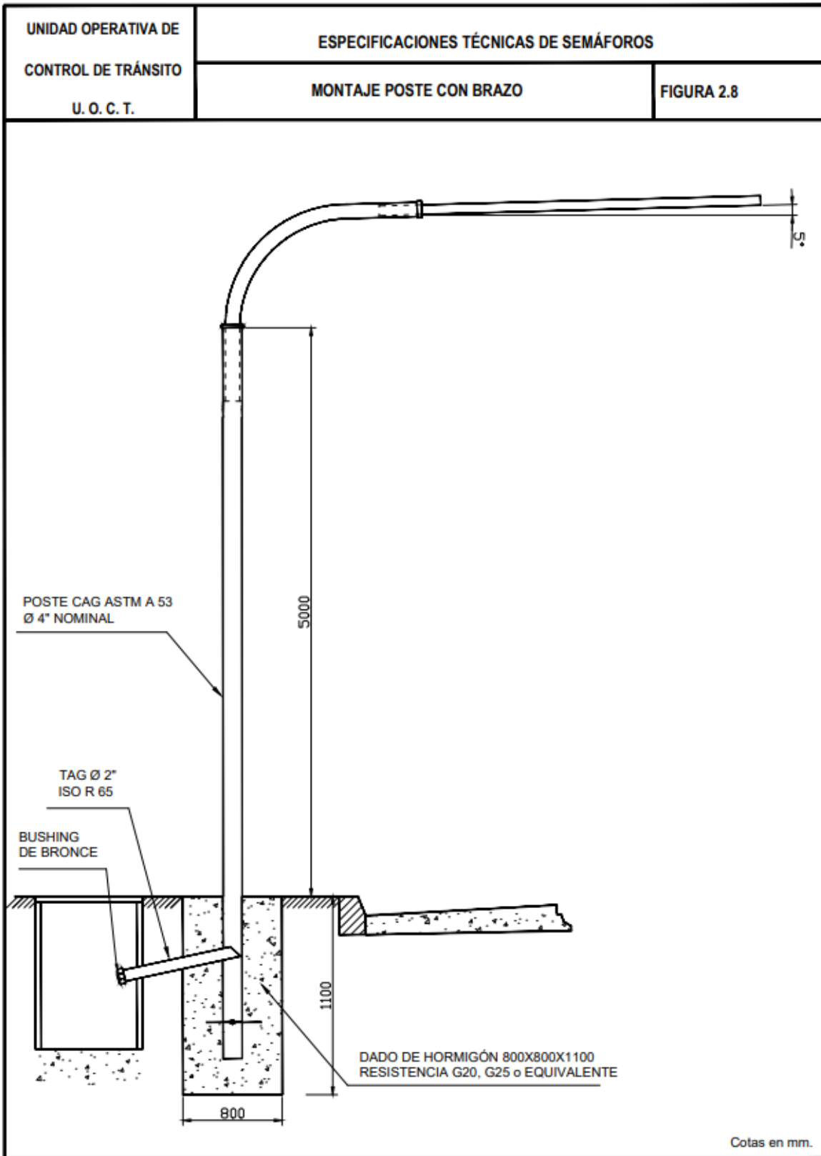
Figura 2. 8 Montaje poste con brazo
