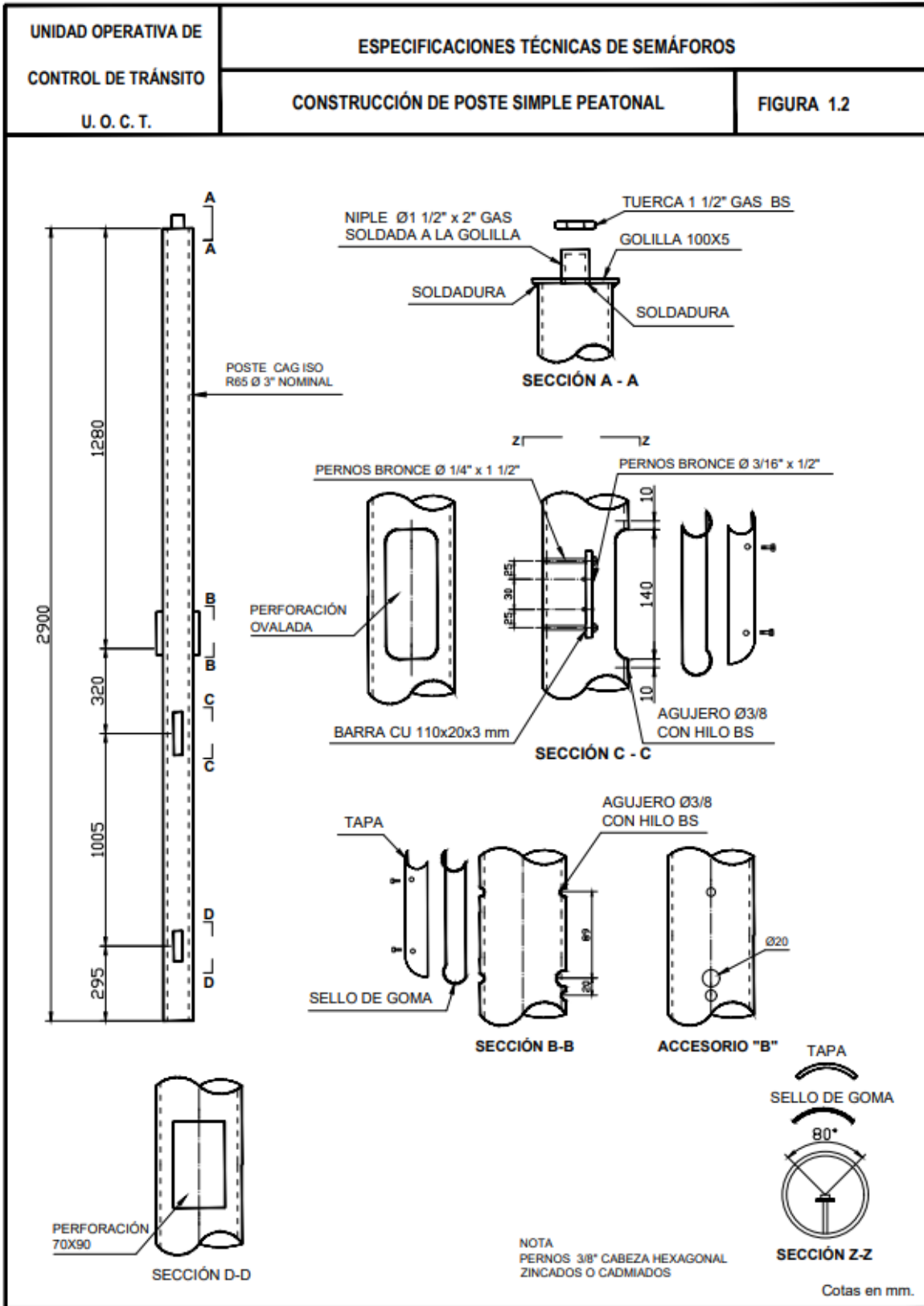
Figura 1. 2 Construcción de poste simple peatonal
