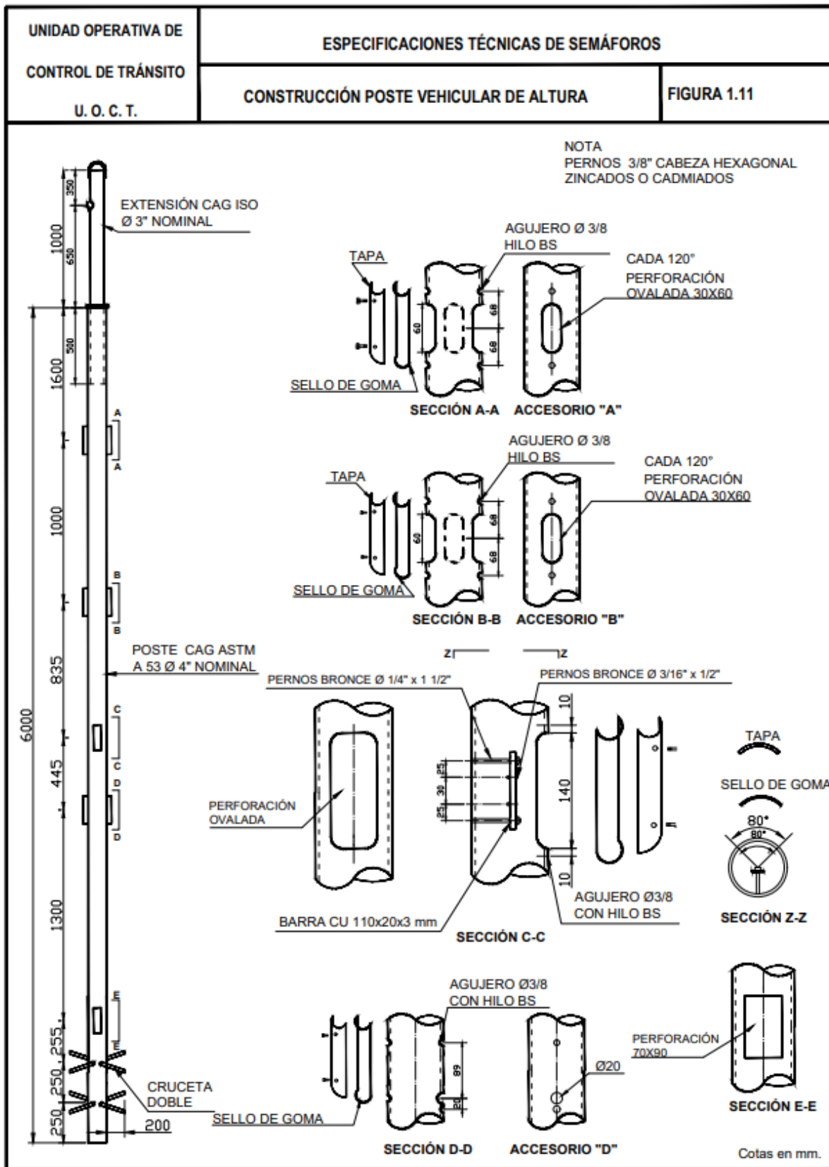
Figura 1. 11 Construcción de Poste Vehicular de altura
