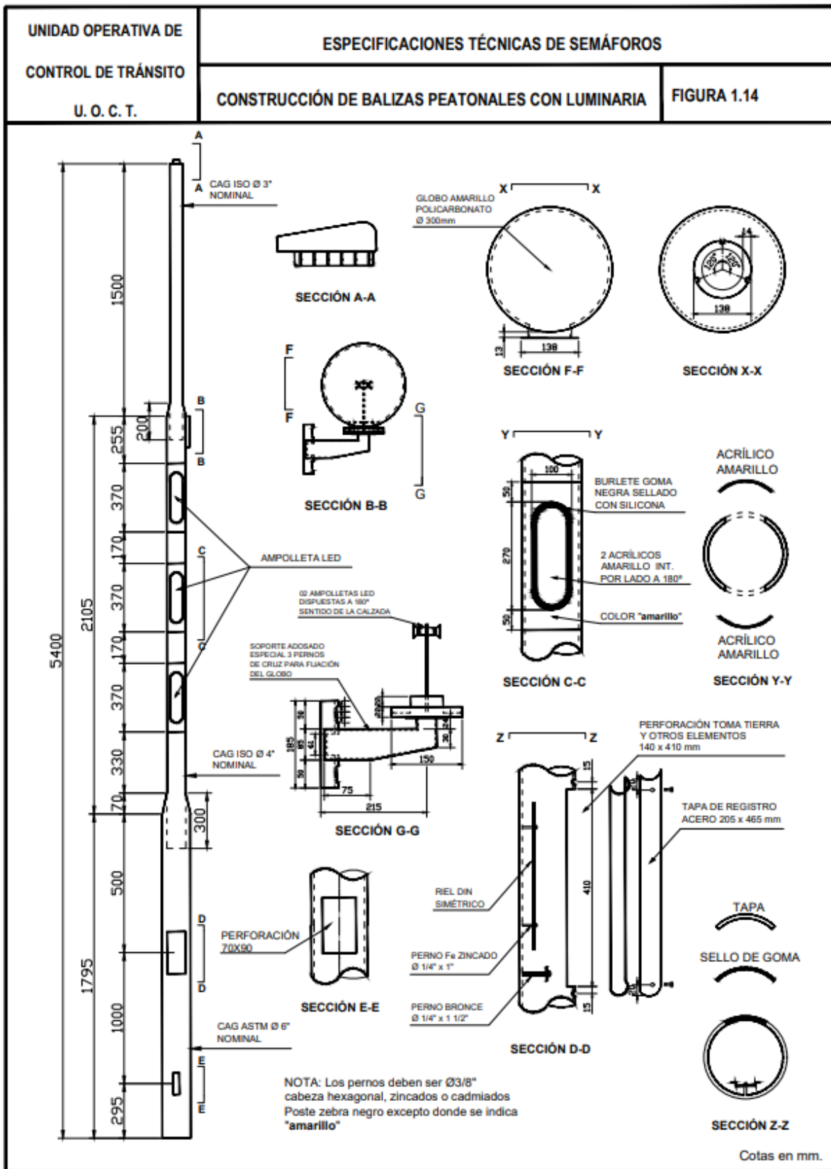
Figura 1. 14 Construcción de balizas peatonales con luminaria
