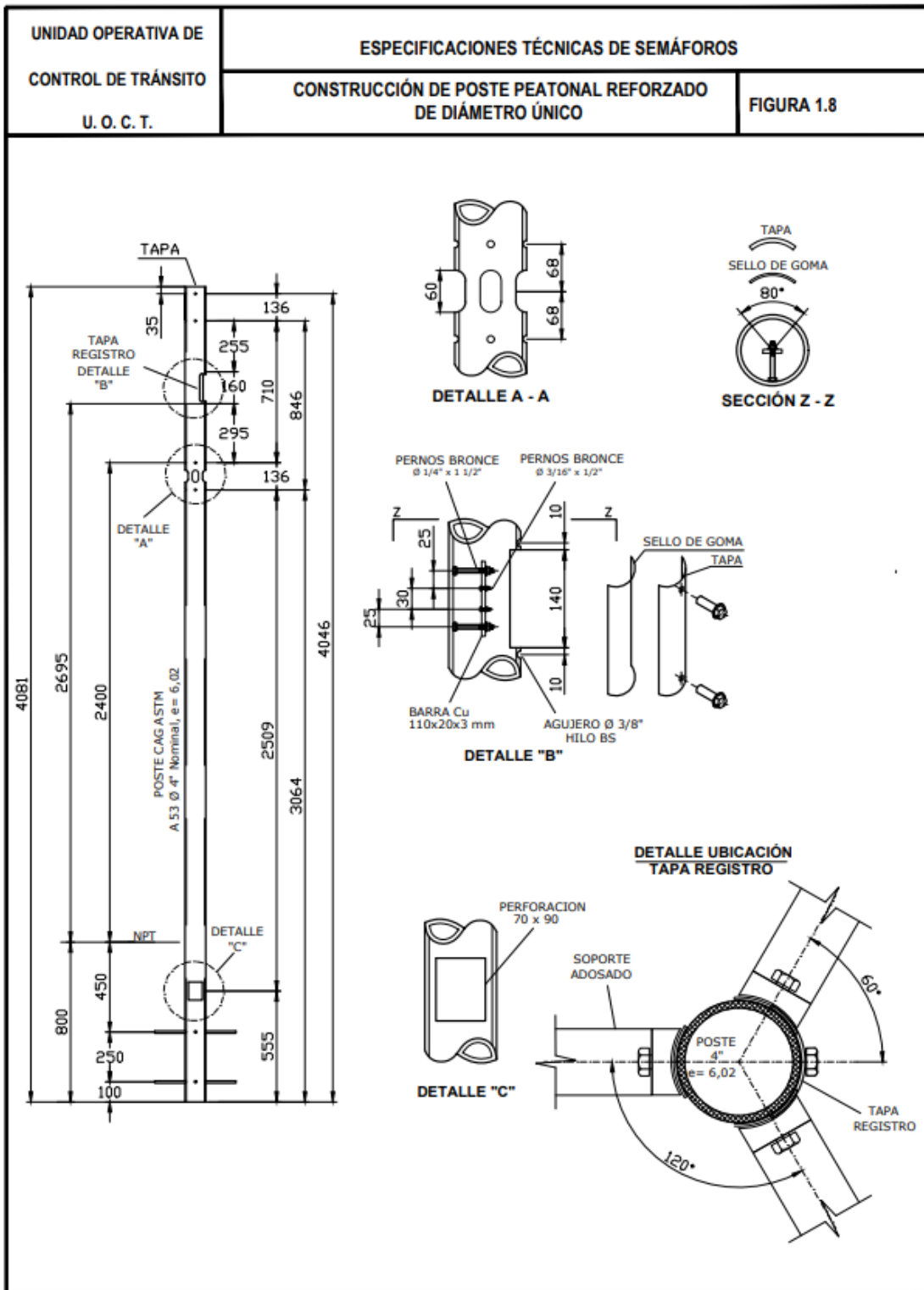
Figura 1. 8 Construcción poste peatonal reforzado de diámetro único
