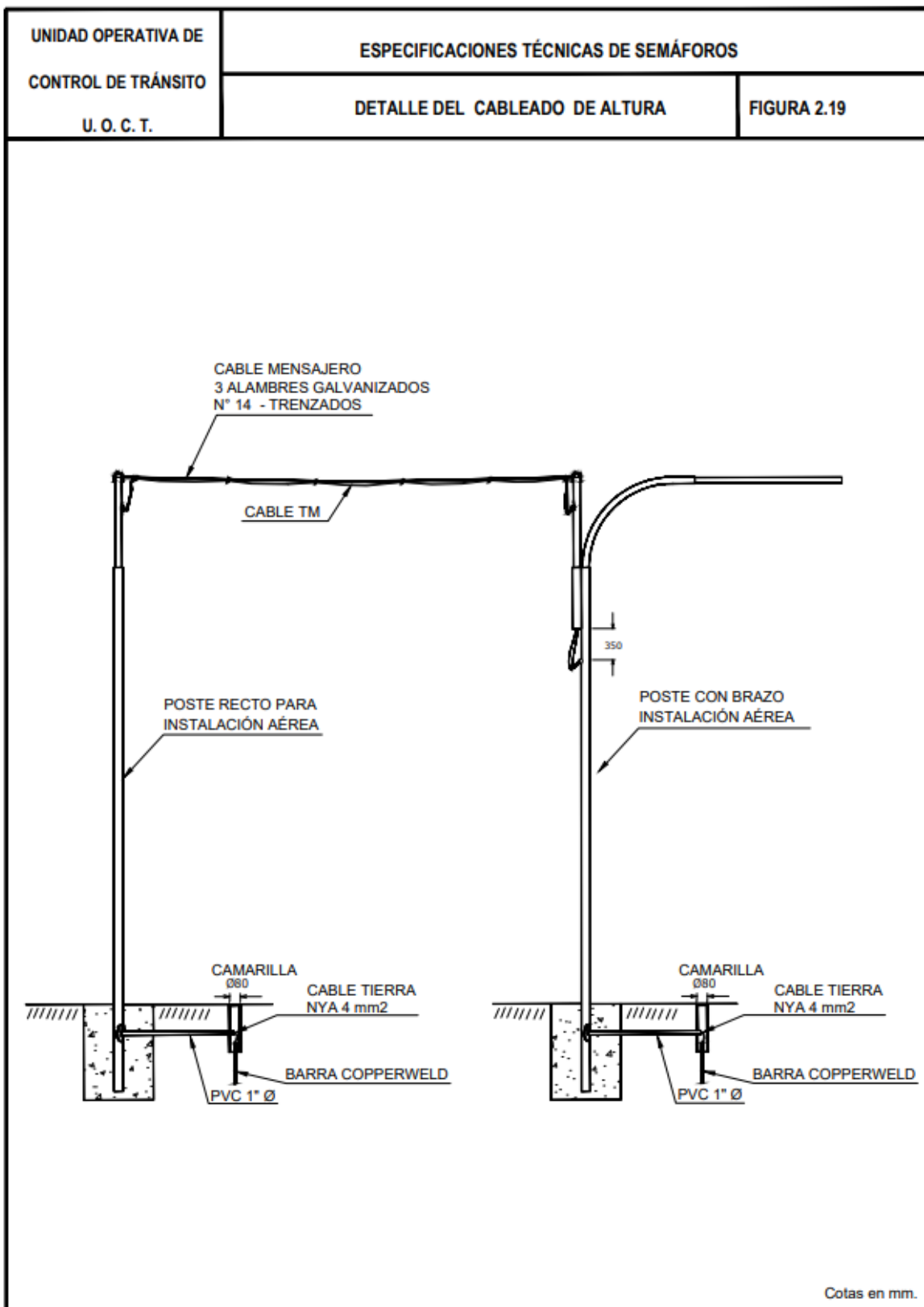
Figura 2. 19 Detalle del cableado de altura
