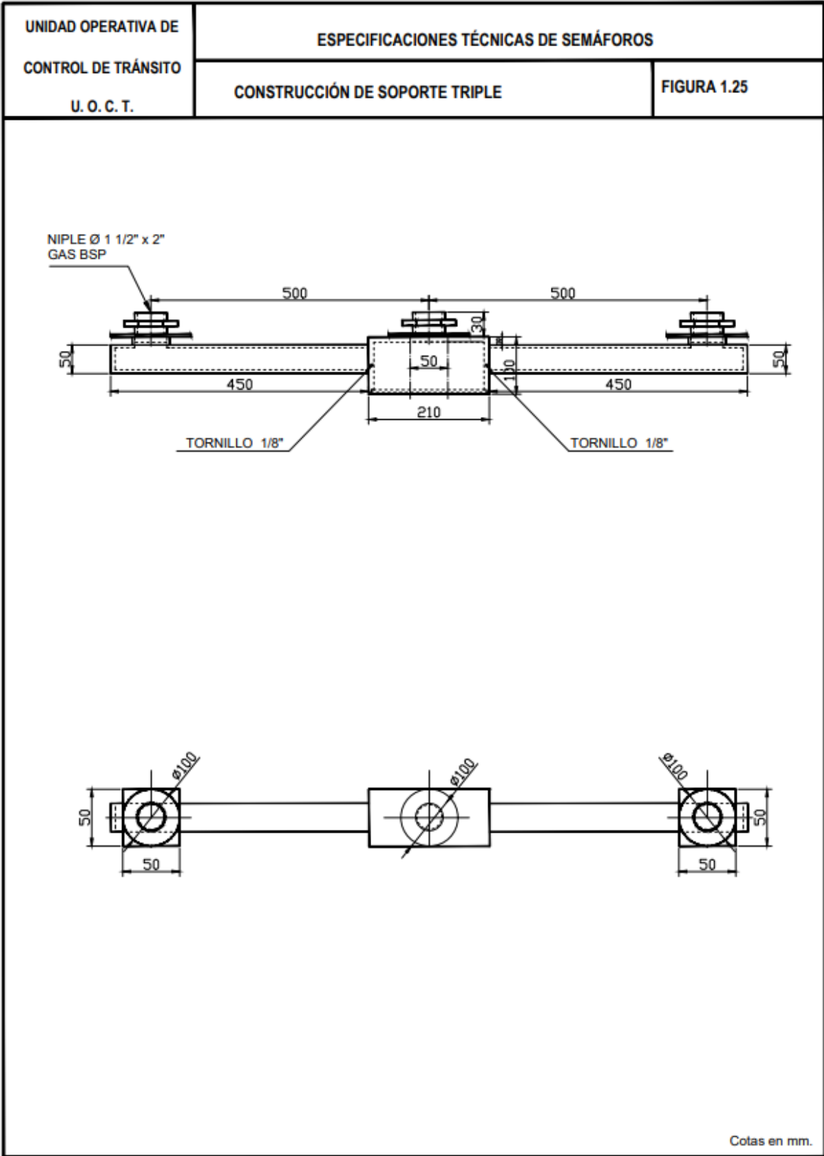
Figura 1. 25 Construcción de soporte triple
