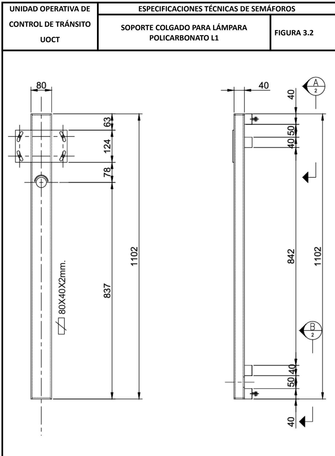
Figura 3. 2 Soporte Colgado para Lámpara de Policarbonato L1
