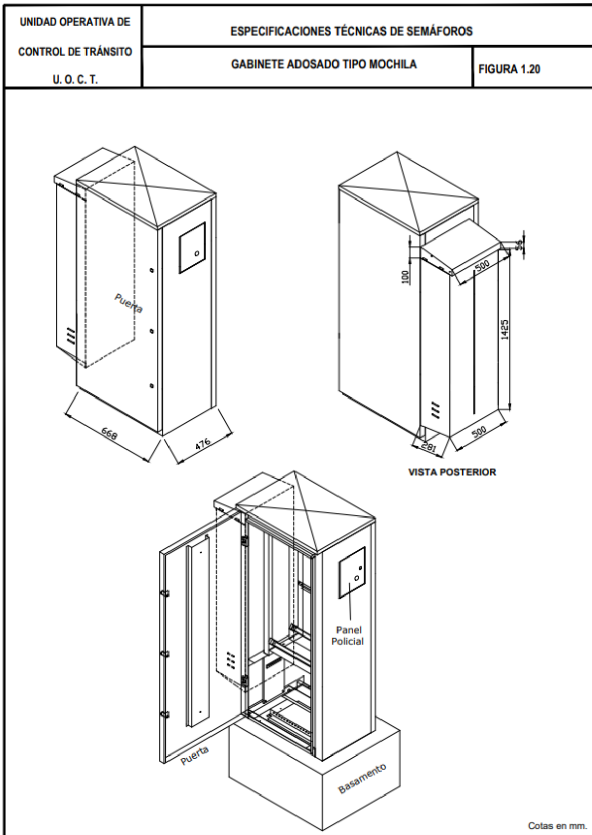
Figura 1. 20 Gabinete adosado tipo mochila
