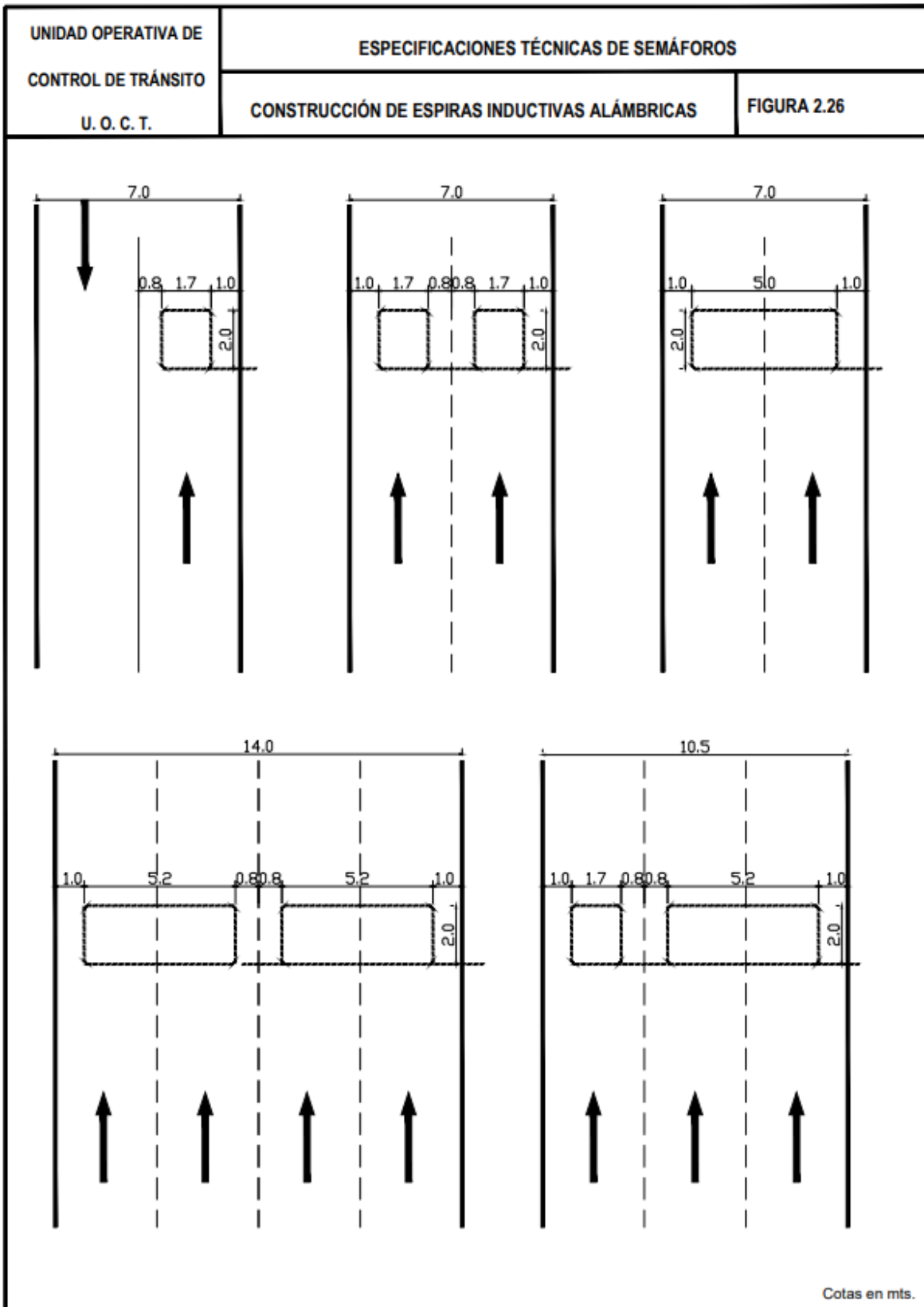
Figura 2. 26 Construcción de espiras inductivas alámbricas
