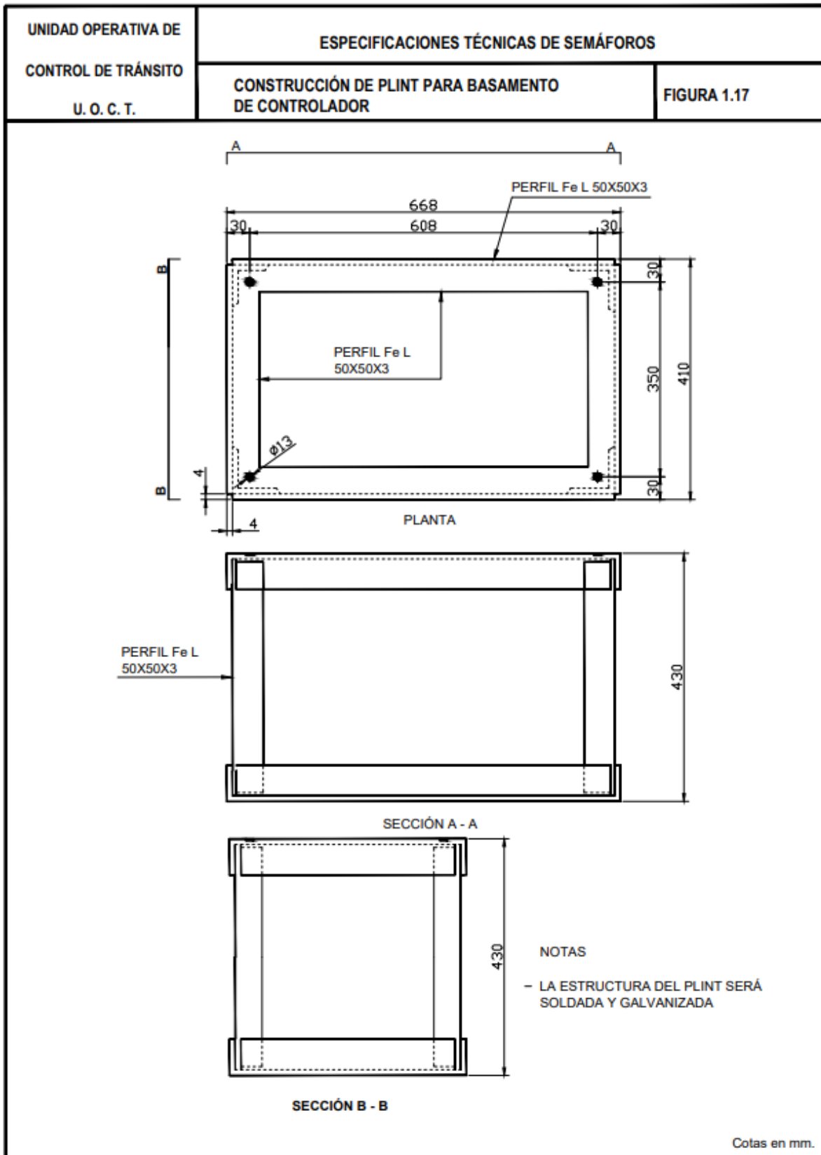
Figura 1. 17 Construcción de Plint para basamento de controlador
