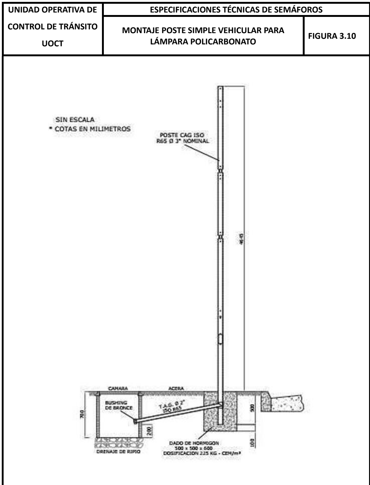
Figura 3.10 Montaje Poste Simple Vehicular para Lámpara de Policarbonato
