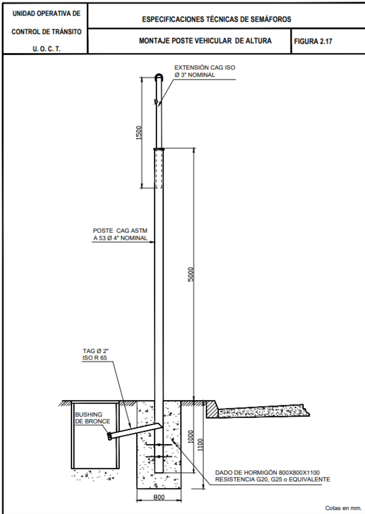
Figura 2. 17 Montaje poste vehicular de altura
