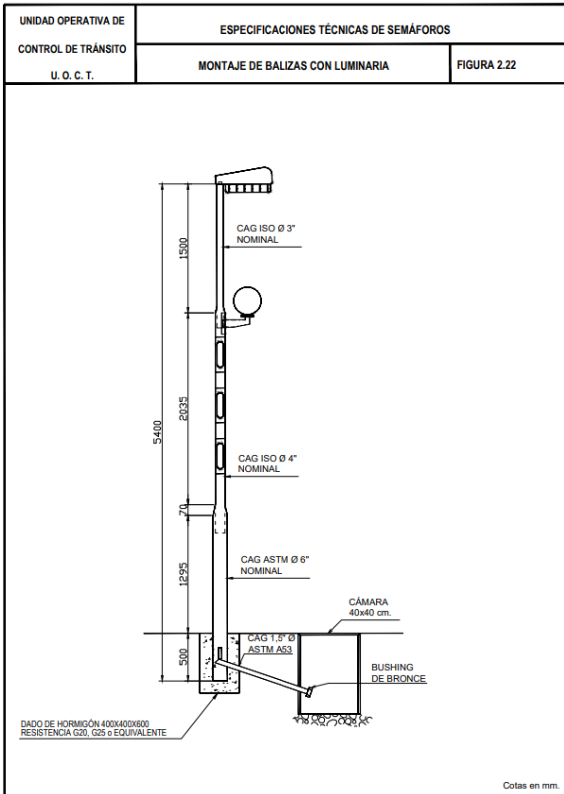
Figura 2. 22 Montaje de balizas con luminaria
