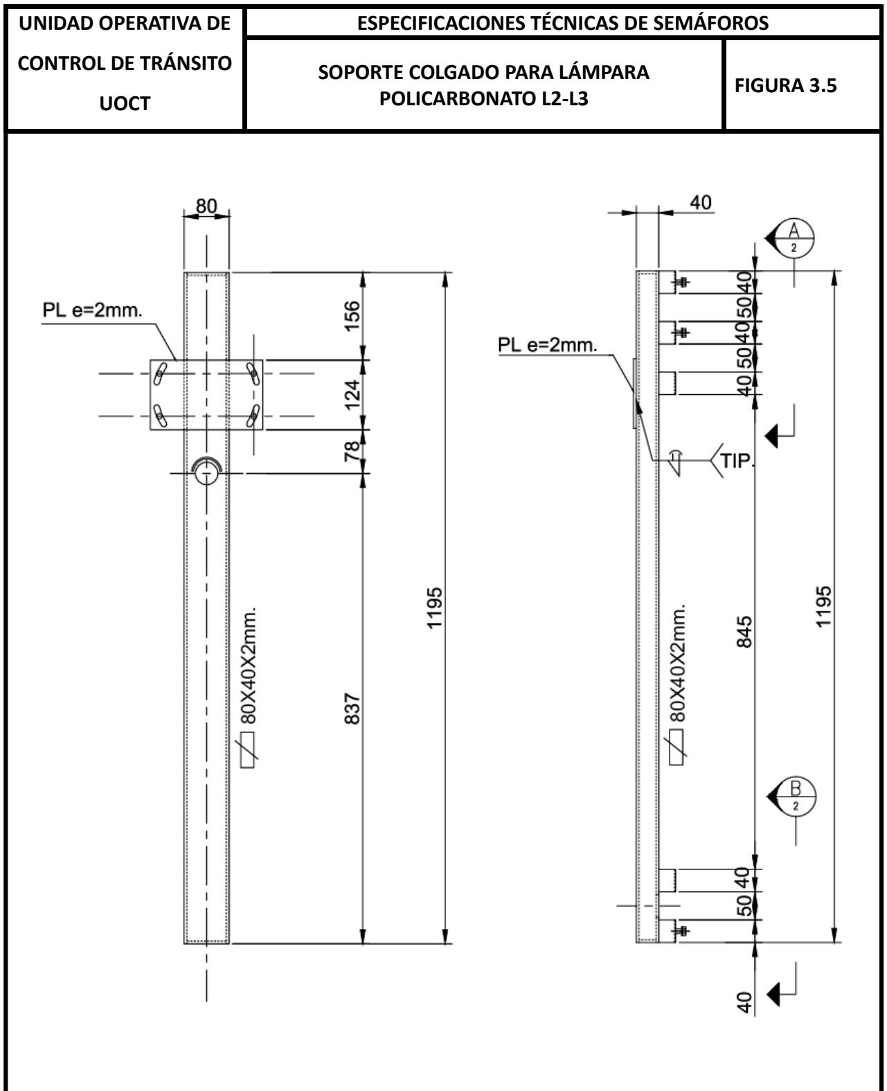
Figura 3. 5 Soporte Colgado Lámparas Policarbonato L1, L2
