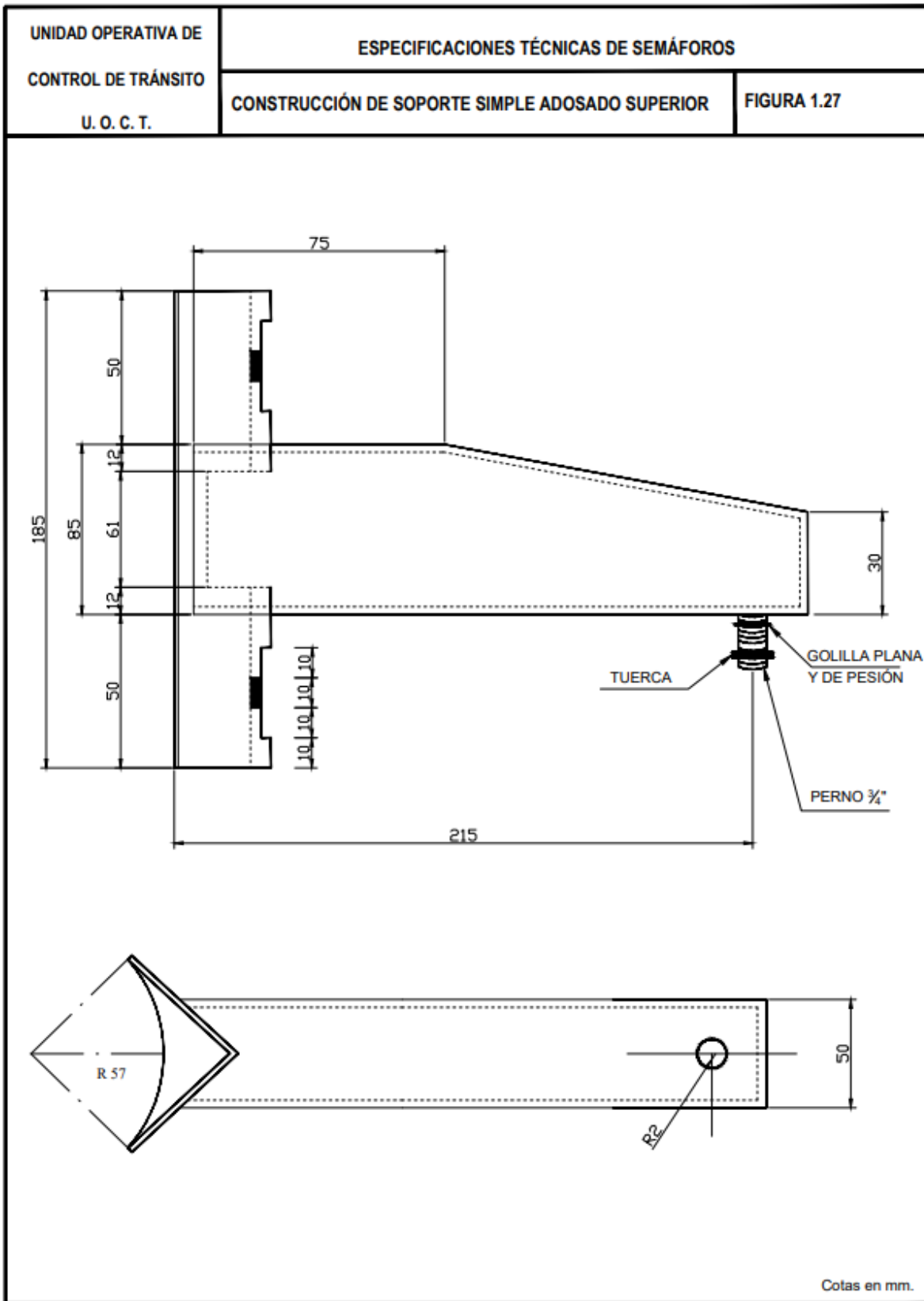
Figura 1. 27 Construcción de soporte simple adosado superior
