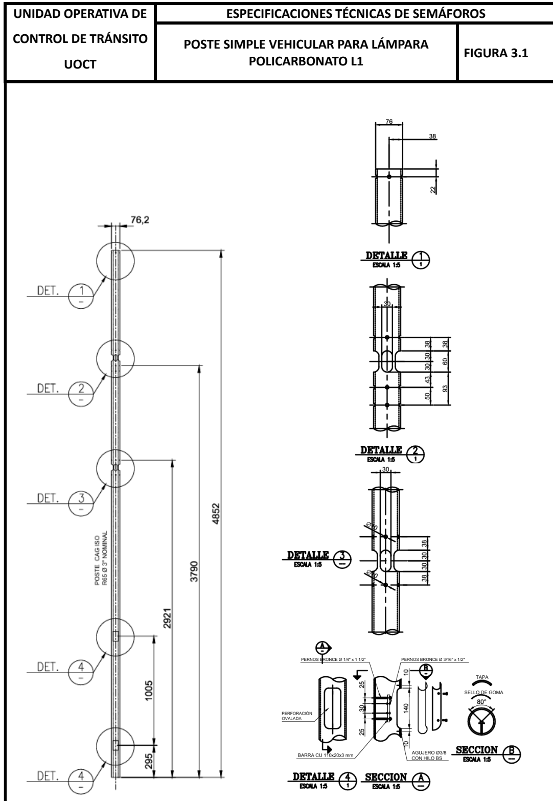
Figura 3. 1 Poste Simple Vehicular L1 para Lámpara de Policarbonato
