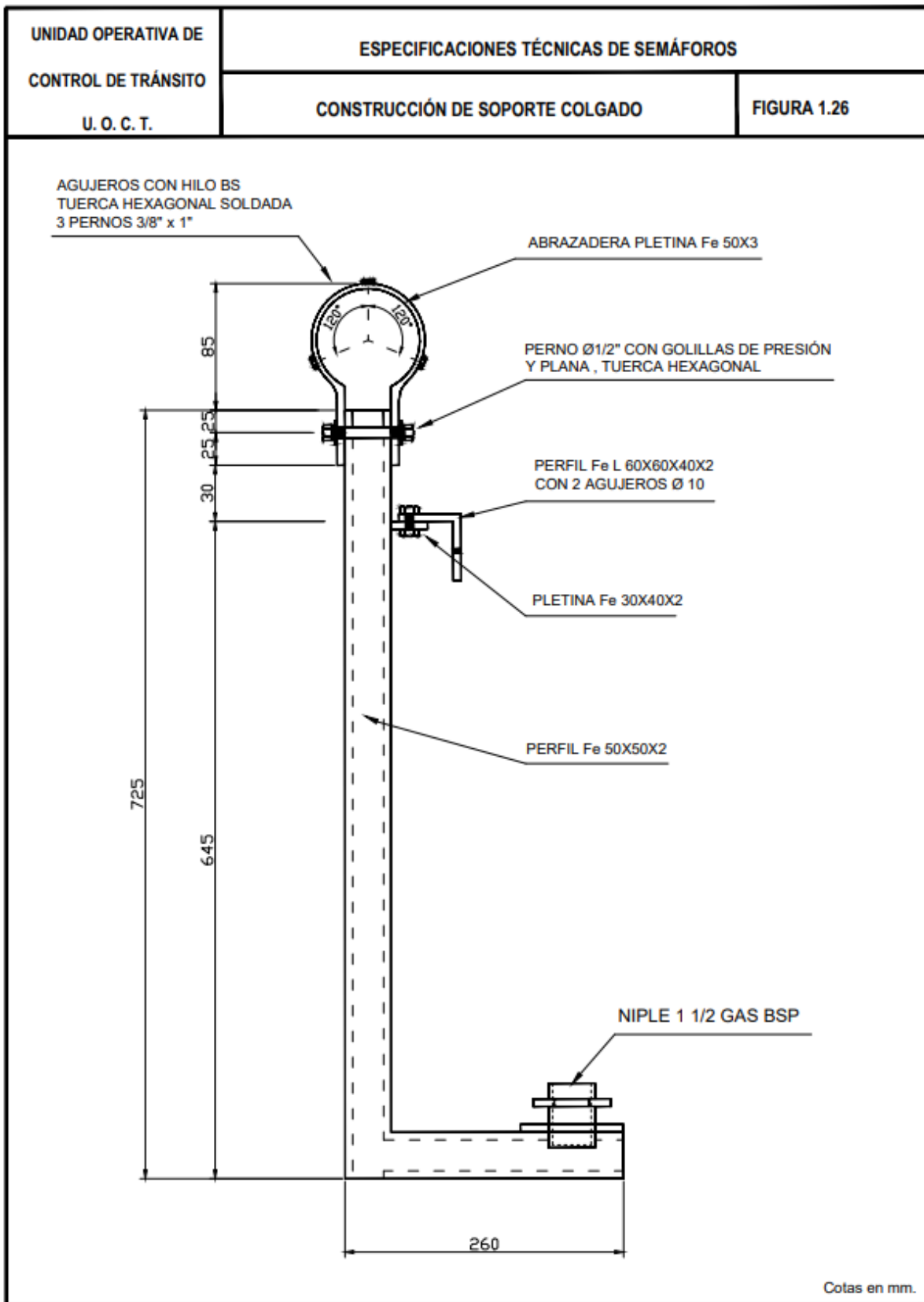
Figura 1. 26 Construcción de soporte colgado
