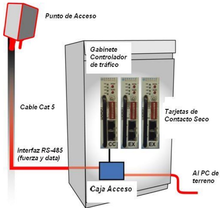
Figura 2. 34 Conexión gabinete
