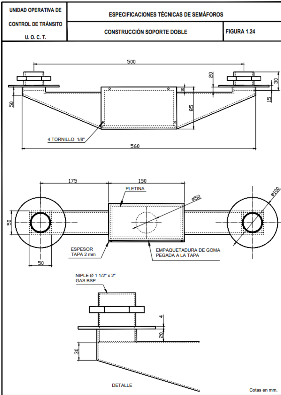
Figura 1. 24 Construcción de soporte doble para lámpara
