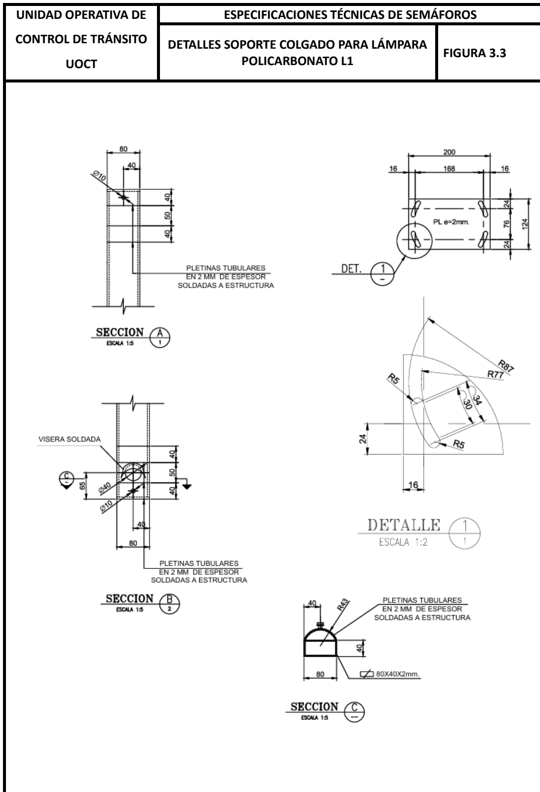
Figura 3. 3 Detalles Soporte Colgado para Lámparas de Policarbonato L1
