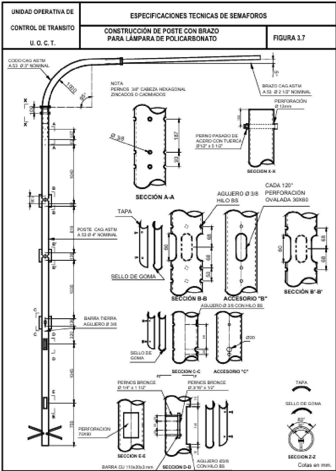
Figura 3.7 Poste con Brazo para Lámpara de Policarbonato
