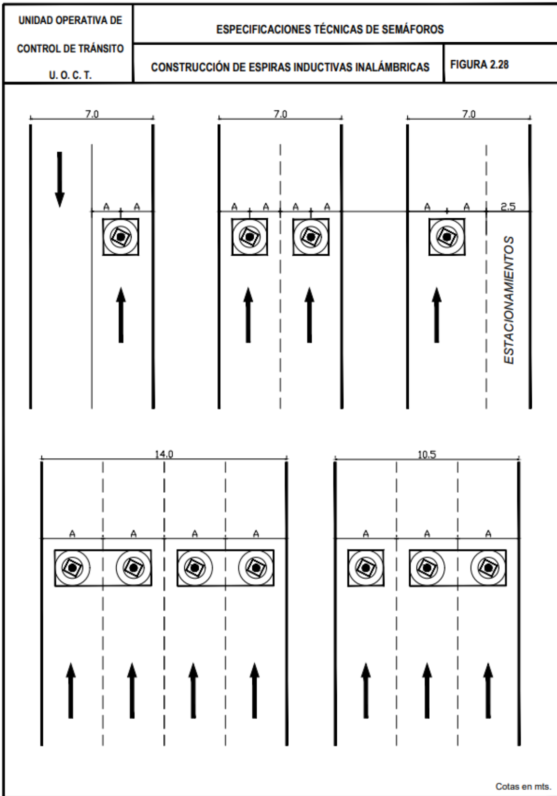
Figura 2. 28 Construcción de espiras inductivas inalámbricas
