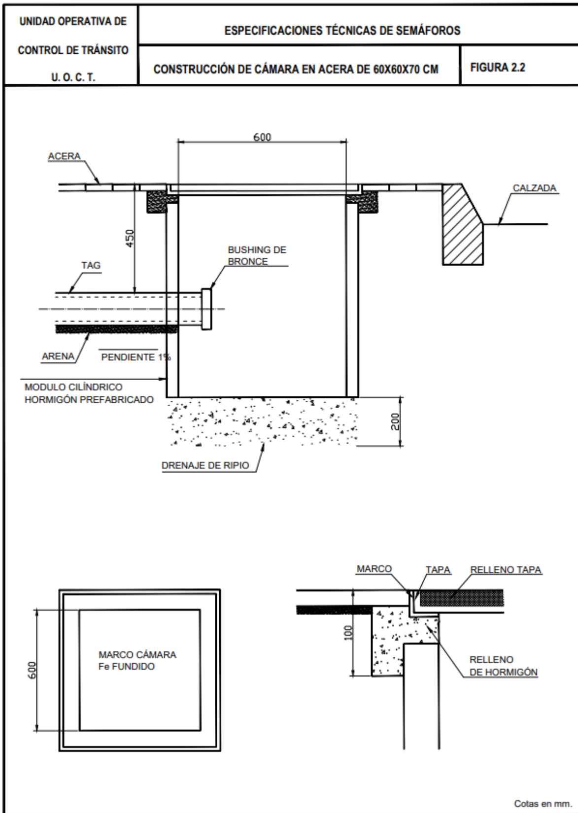
Figura 2. 2 Construcción de cámara en acera de 60x60x70 cm
