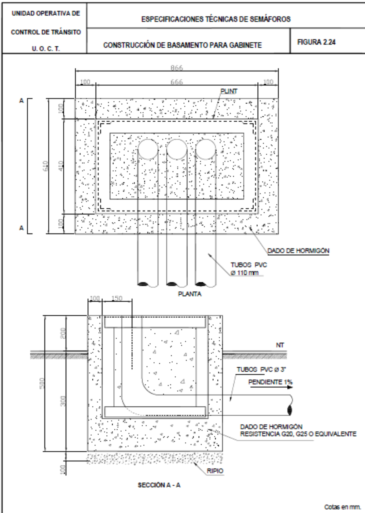
Figura 2. 24 Construcción de basamento para controlador, CCTV y UPS
