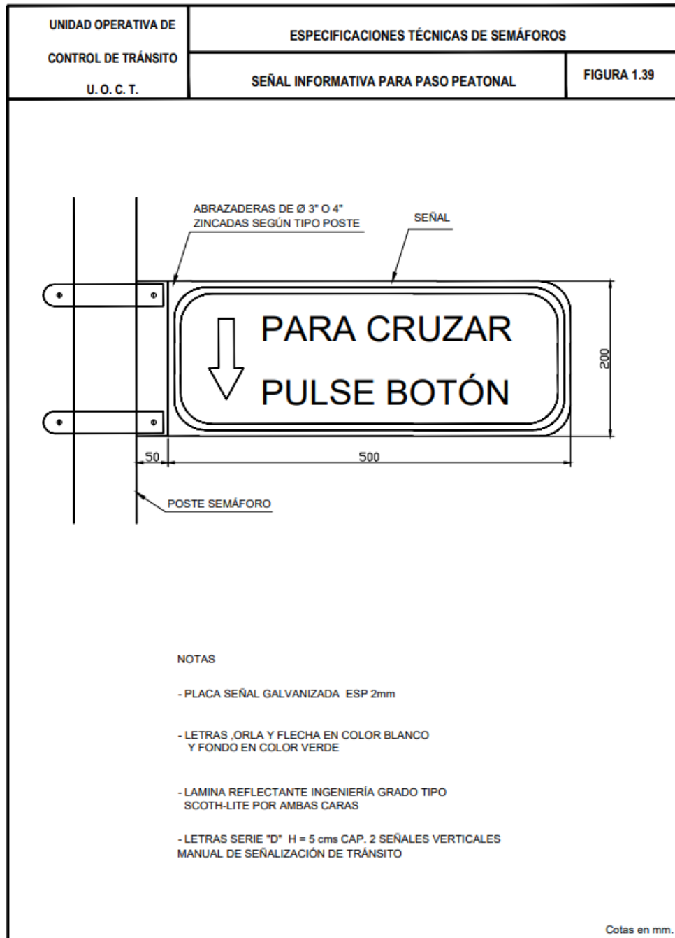
Figura 1. 39 Señal informativa para paso peatonal
