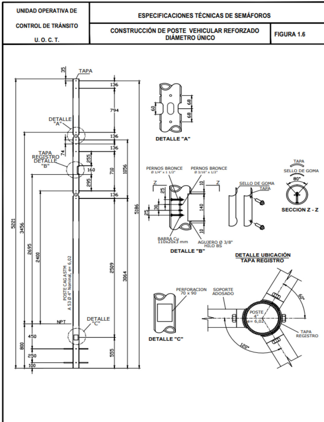
Figura 1. 6 Construcción de poste simple peatonal reforzado diámetro único
