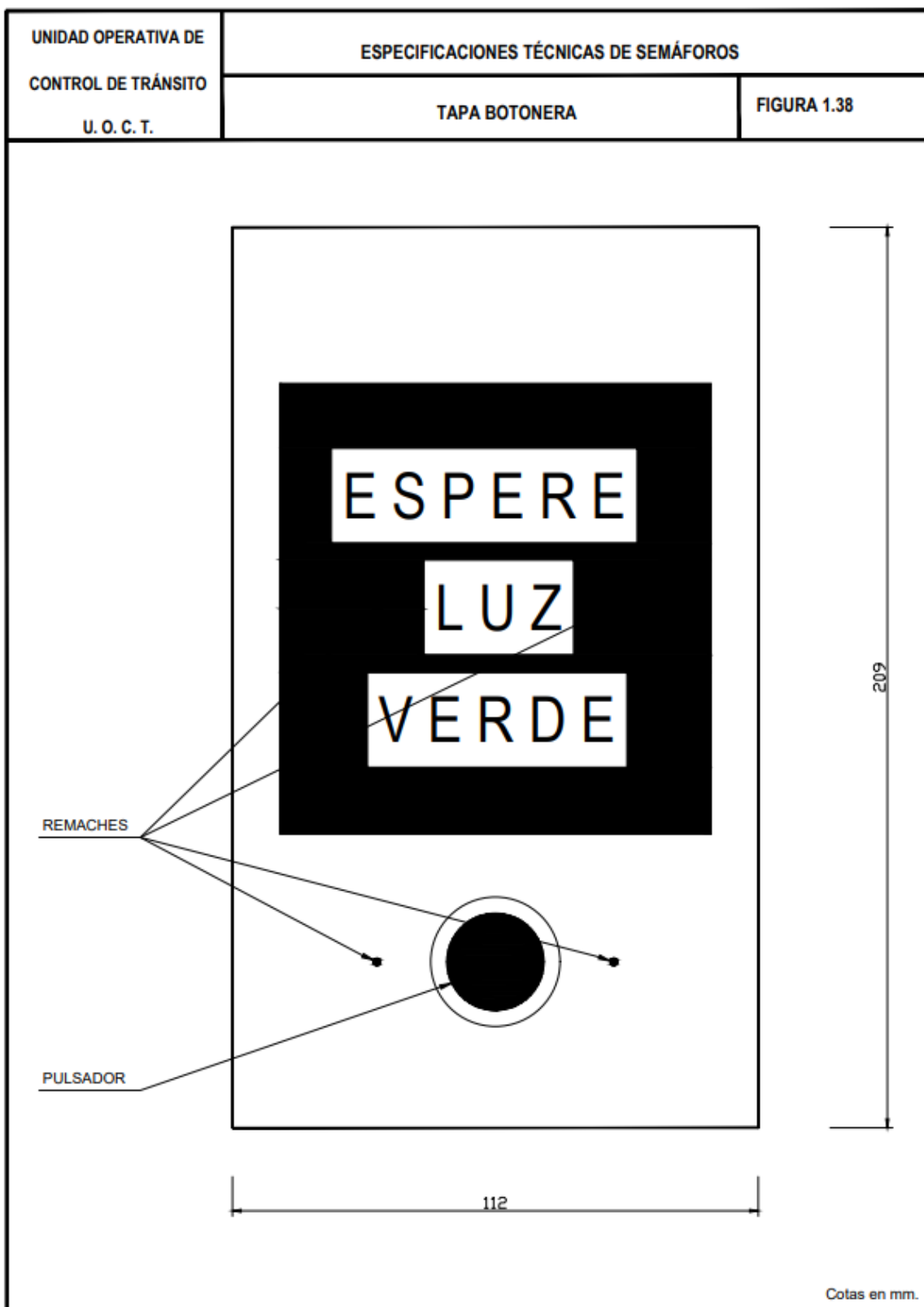
Figura 1. 38 Tapa botonera
