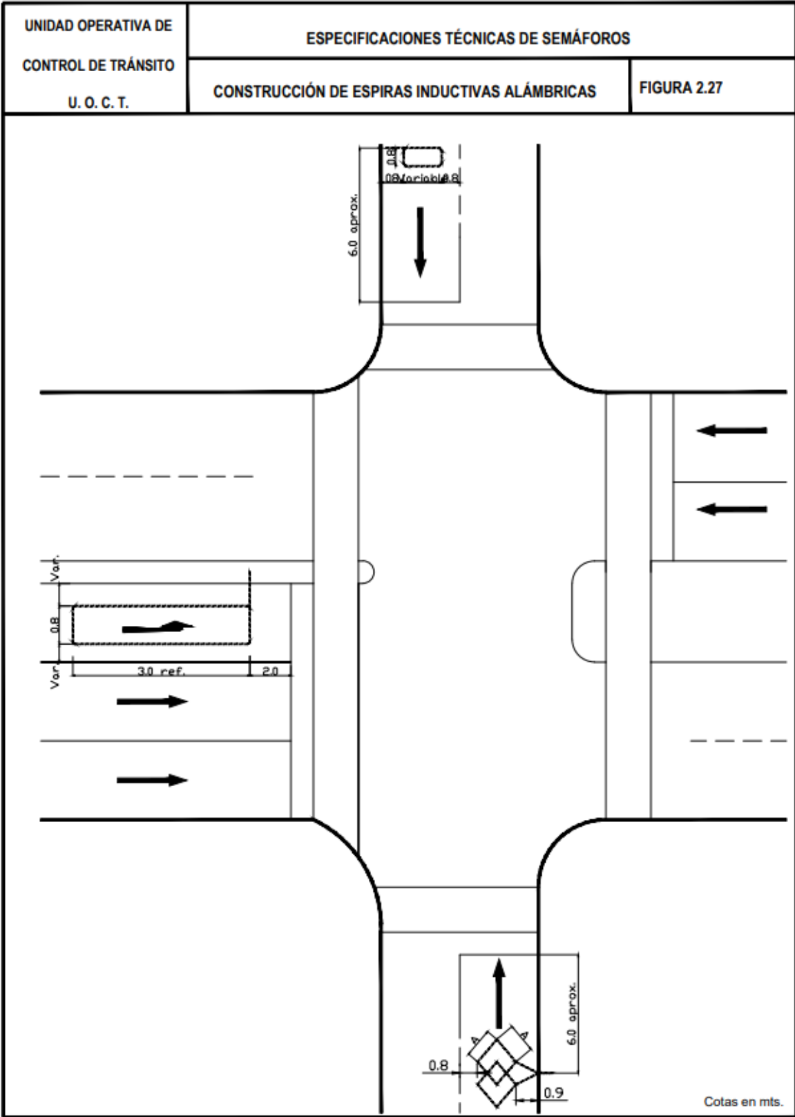
Figura 2. 27 Construcción de espiras inductivas alámbricas B
