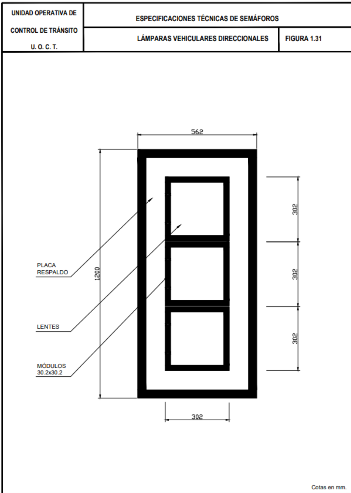
Figura 1. 31 Lámparas vehicular direccional
