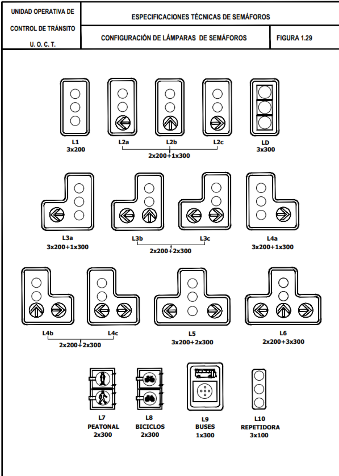
Figura 1. 29 Configuración de lámparas de semáforos
