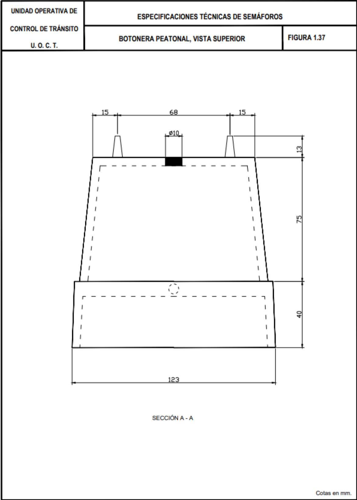
Figura 1. 37 Botonera peatonal, vista superior
