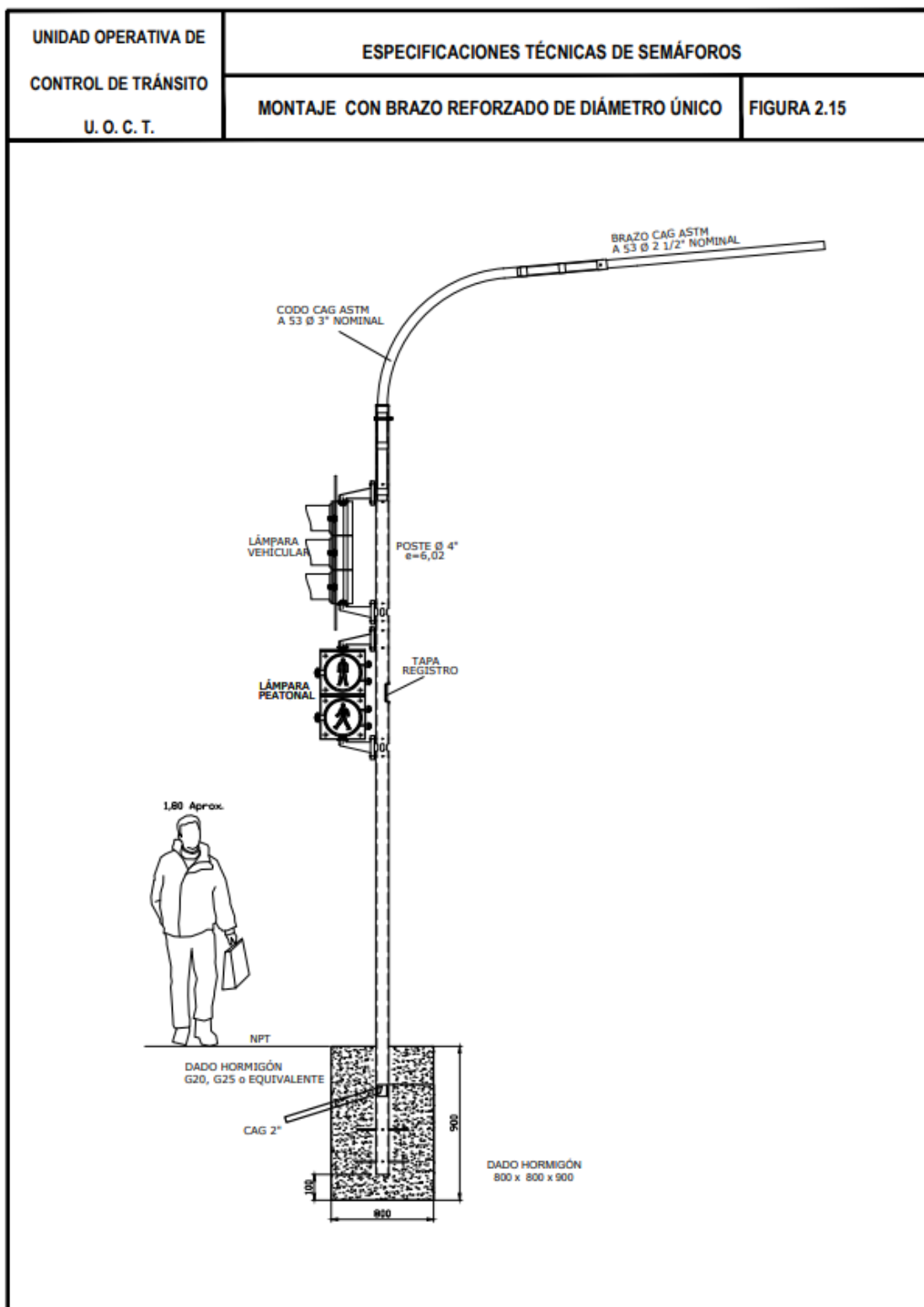
Figura 2. 15 Montaje con brazo reforzado de diámetro único
