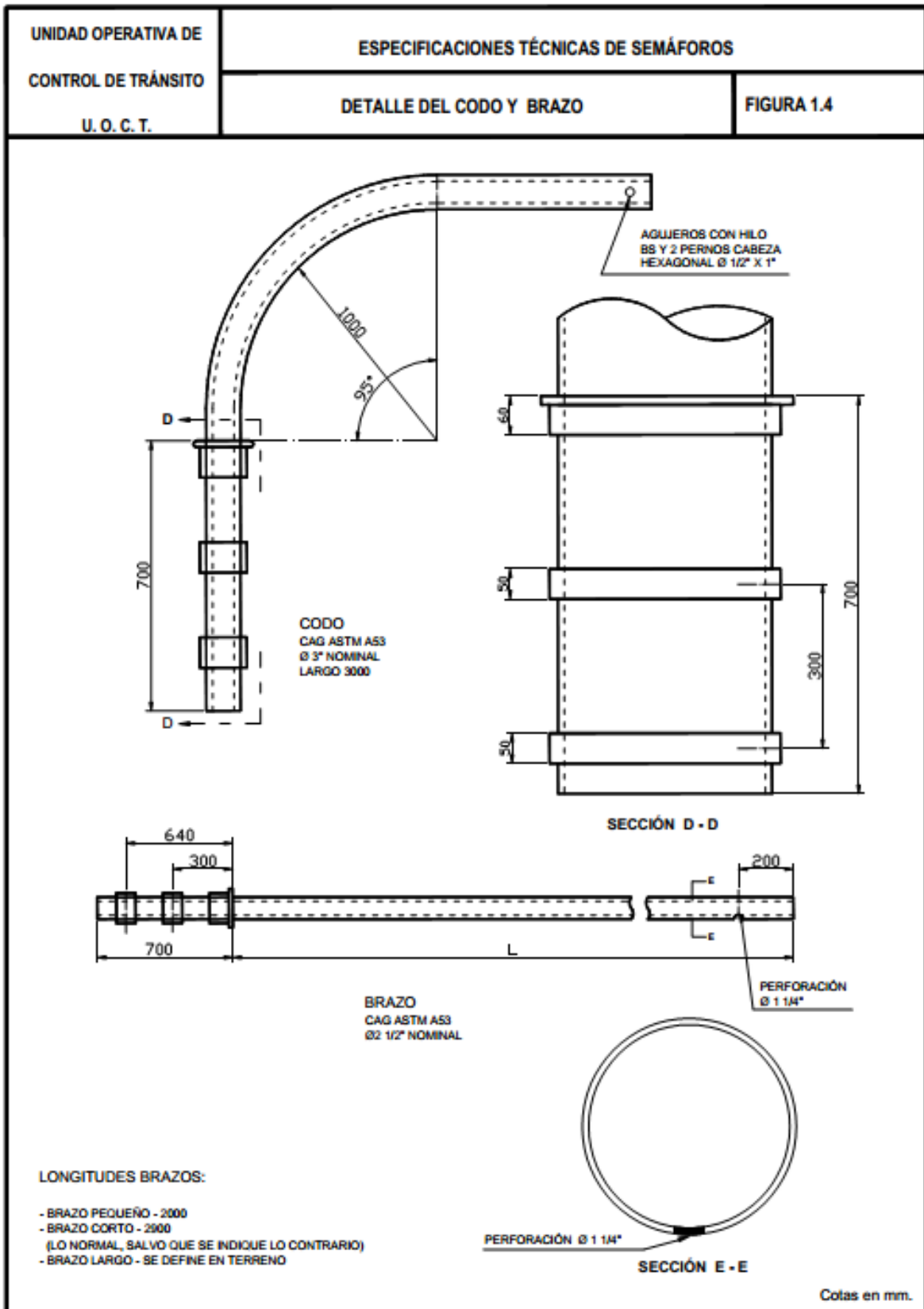
Figura 1. 4 Detalle del codo y brazo
