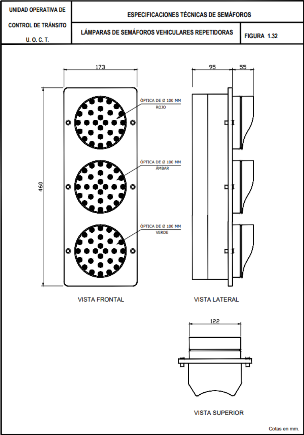
Figura 1. 32 Lámparas de semáforos vehiculares repetidoras
