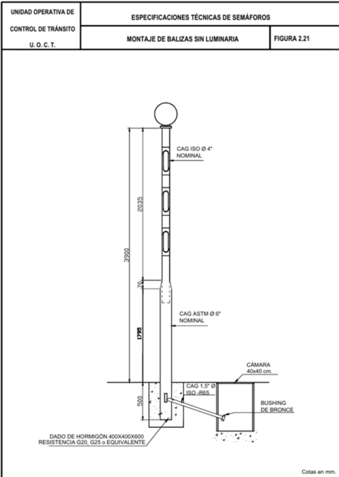
Figura 2. 21 Montaje de balizas sin luminaria
