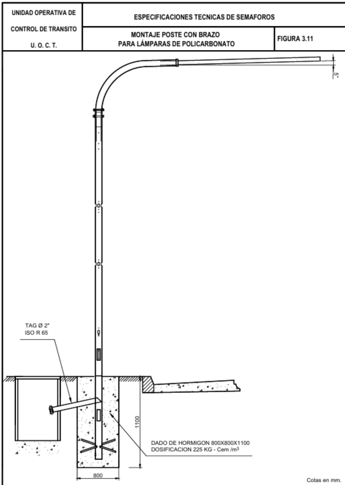
Figura 3. 11 Montaje Poste con Brazo Lámpara de Policarbonato
